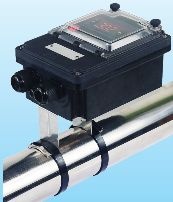
在垂直管道上带有背面安装支架选项的安装示例
