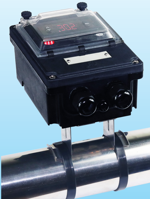
在水平管道上带有背面安装支架选项的安装示例
